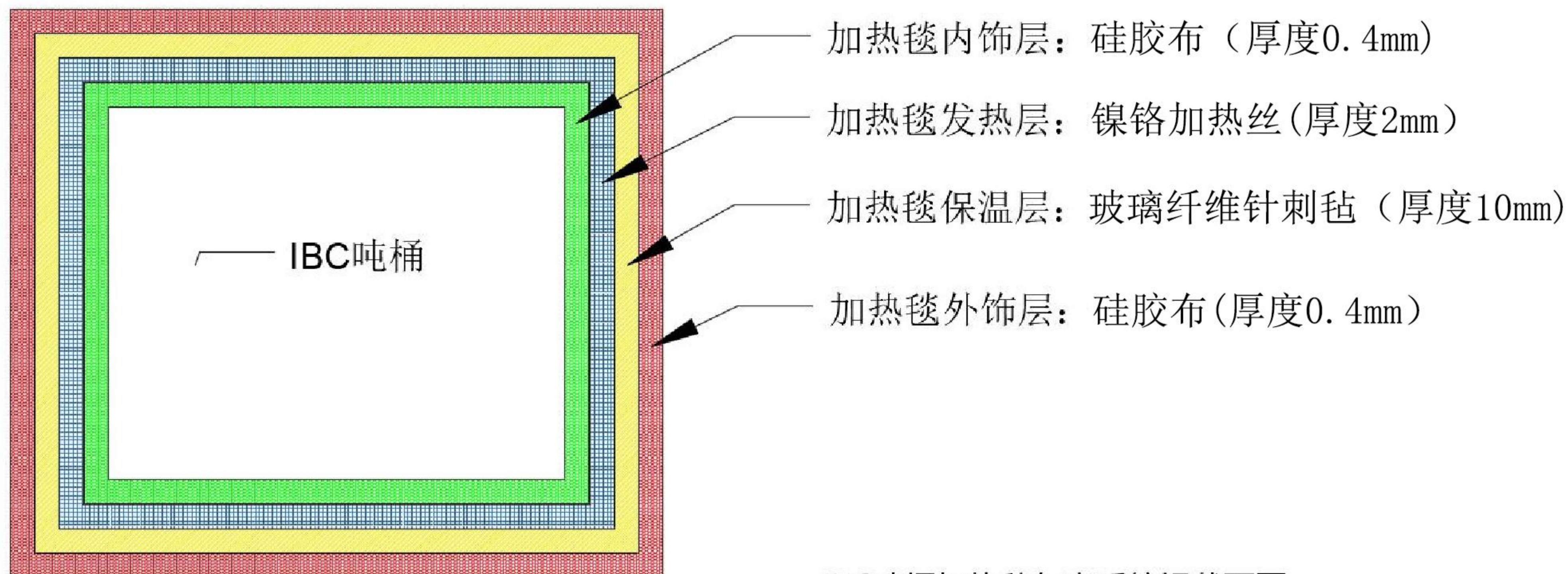
IBC吨桶加热毯包裹后俯视截面图
